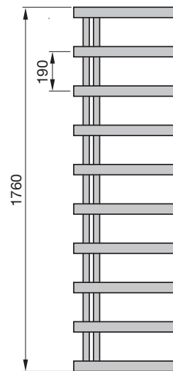
Pohled zepředu CHZ-180-050
