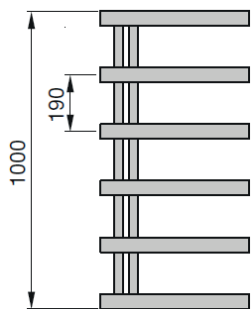
Pohled zepředu CHZ-100-050
