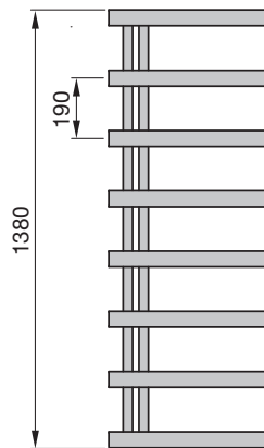
Pohled zepředu CHZ-140-050
